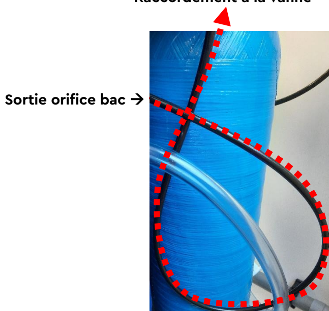
Raccordement à la vanne
